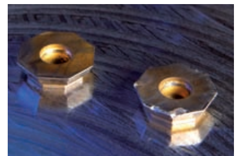
Schneidplatten: links mit ES Antikor SL bearbeitet, rechts mit herkömmlichem Stahl
